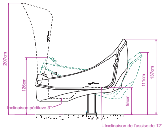
CUVE EN POSITION HAUTE SANS PIÉTEMENT
